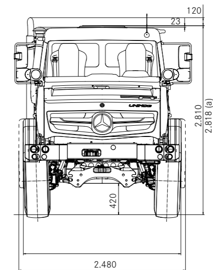
(a) Unbeladenes Fahrzeug Darstellung im eingefederten Zustand, mit Bereifung 365/85 R 20, mit SA = Sonderausstattungen, alle Maße in mm.
