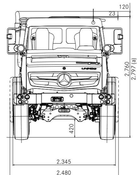
(a) Unbeladenes Fahrzeug Darstellung im eingefederten Zustand, mit Bereifung 335/80 R 20, mit SA = Sonderausstattungen, alle Maße in mm.
