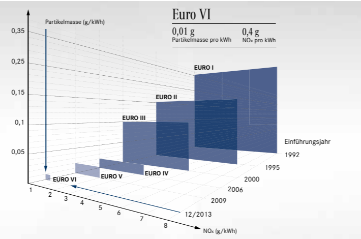
Mehr Leistung, weniger Emissionen: Der BlueTec 6-Motor leistet beim hochgeländegängigen Unimog als 4-Zylinder-Aggregat 170 kW. Das moderne Triebwerk erfüllt in Verbindung mit dem Kühlsystem und der Abgasnachbehandlungsbox die Abgasnorm Euro VI. Sie verlangt eine Reduktion von Dieselpartikel- und Stickoxidemissionen um 90% gegenüber Euro V.
