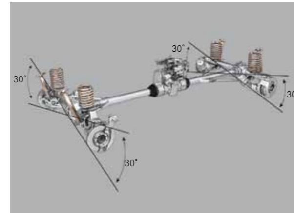
Schubrohrtechnik und Schraubfedern ermöglichen extreme Federwege und eine große Achsver-schränkung bis zu 30°.
