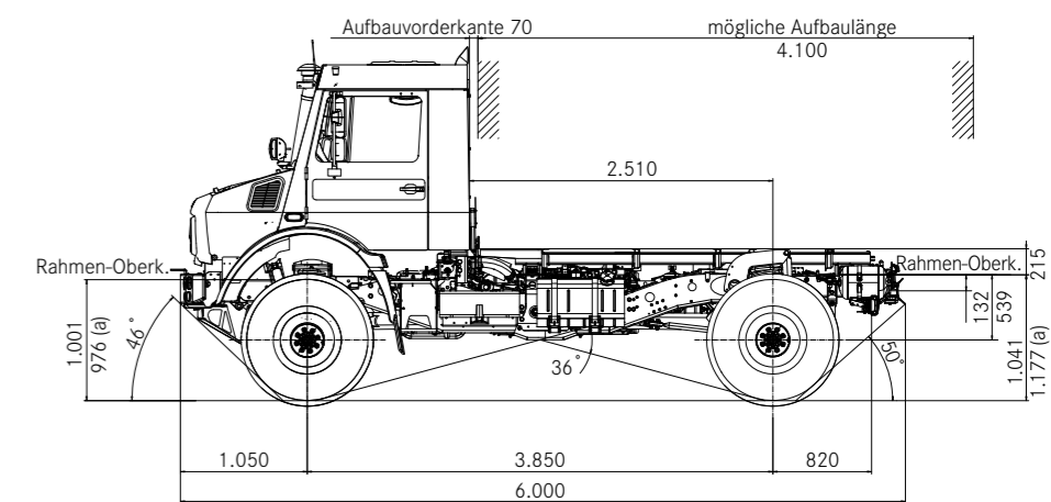
(a) Unbeladenes Fahrzeug Darstellung im eingefederten Zustand, mit Bereifung 365/85 R 20, mit SA = Sonderausstattungen, alle Maße in mm.
